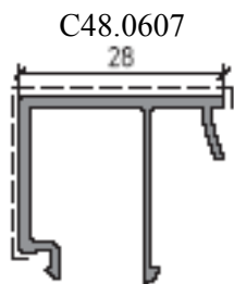
Штапик 28 мм
