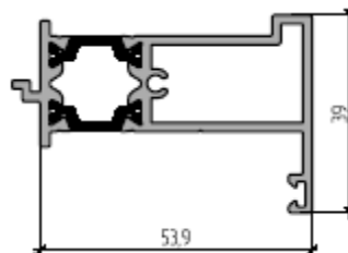
Штульп 39 мм
