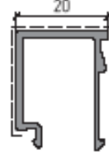
Штапик 20 мм
