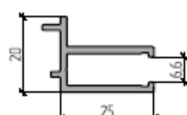
Профиль термоком- пенсационный 20 мм
