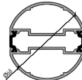
Соединитель «труба» 68 мм
