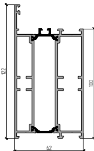
Рама 100/122 мм
