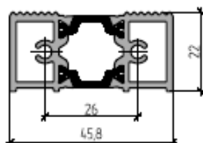
Порог 22 мм теплый
