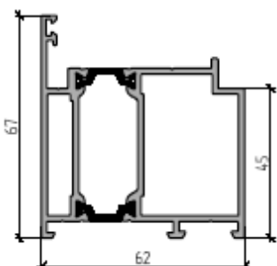
Рама компланарная 45/67 мм внутреннего открывания
