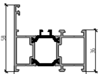
Рама 36/58 мм
