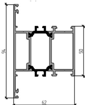
Импост 50/94 мм W62.0801
