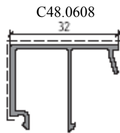
Штапик 32 мм
