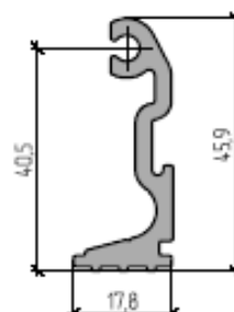
Профиль крепления импоста
