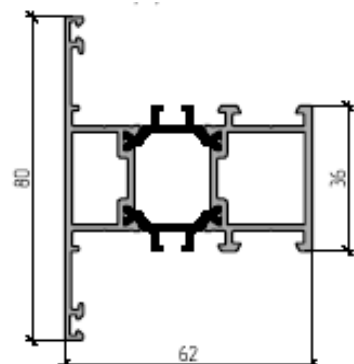
Импост 36/80 мм
