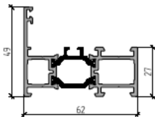
Рама 27/49 мм
