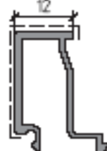
Штапик 12 мм
