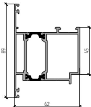
Створка компланарная Т-обр. 45/89 мм наружного открывания
