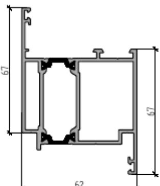
Створка компланарная Z-обр. 67/89 мм внутреннего открывания
