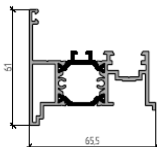
Штульп 61 мм
