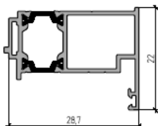
Профиль дверной вспомогательный 22 мм
