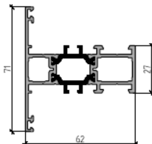
Импост 27/71 мм
