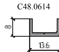
Профиль выравнивающий
