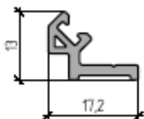
Клипса «трубы» внутренняя
