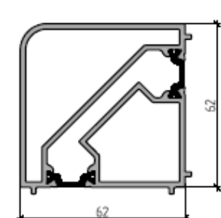
Соединитель 90 град.
