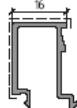
Штапик 16 мм
