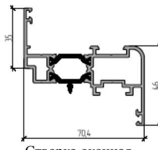
Створка оконная 46/68 мм
